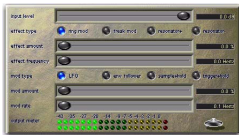
Sci-Fi
